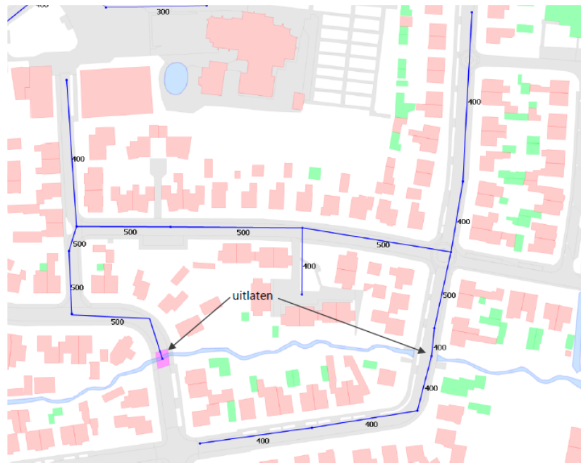
Figuur 2. Voorgesteld HWA-stelsel
